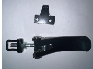
U-910/911 Gancho troperzon chico/grande (negro)
